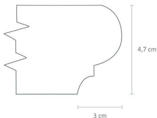
GRADINO CON CORNICE - SEZIONE BULLNOSE STEPS - PROFILE
